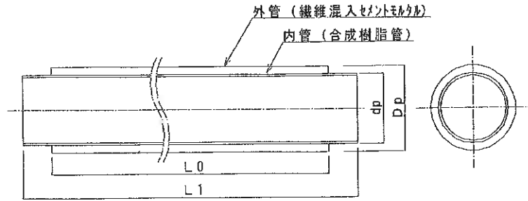
図-2 耐火二層管寸法図
