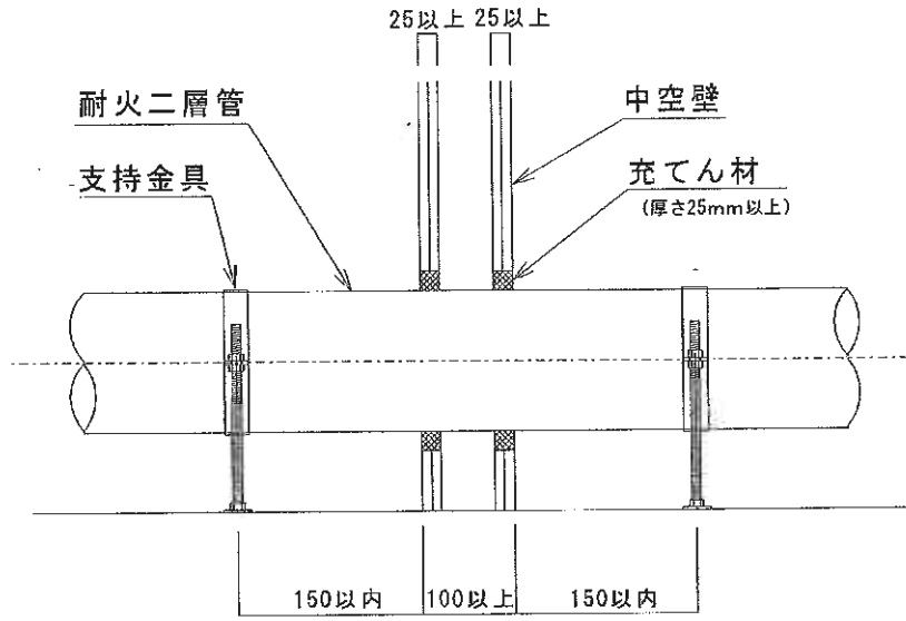
図-5 埋め戻しと配管支持
