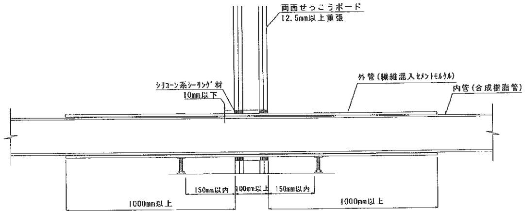
断面図
