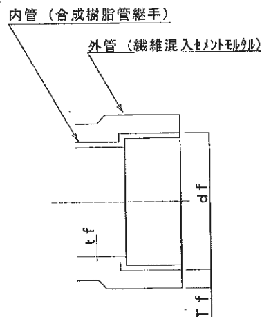
図-3 管継手の受け口形状・寸法図
